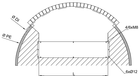
System mocowania
