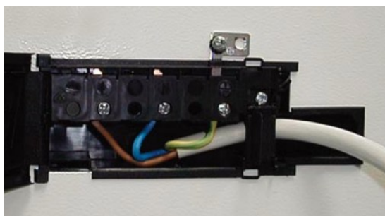
Zaciski przyłączeniowe kurтын „zimnych”: L, N i uziemienie (230 V) dla zasilania wentylatorów.
