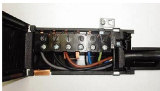
Puszka podłączeniowa kurтын elektrycznych: zaciski 2, 3, 4 (380 V) dla zasilania grzałek oraz L, N (230 V) i uziemienie dla zasilania wentylatorów.
