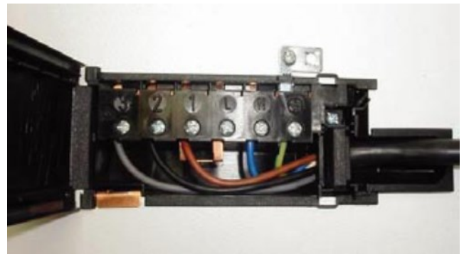
Puszka podłączeniowa kurtyn elektrycznych: zaciski 2, 3, 4 (380 V) dla zasilania grzałek oraz L, N (230 V) i uziemienie dla zasilania wentylatorów.
